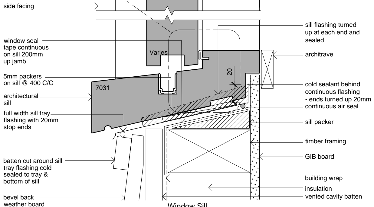
Window Sill Scale: 1:2.5
