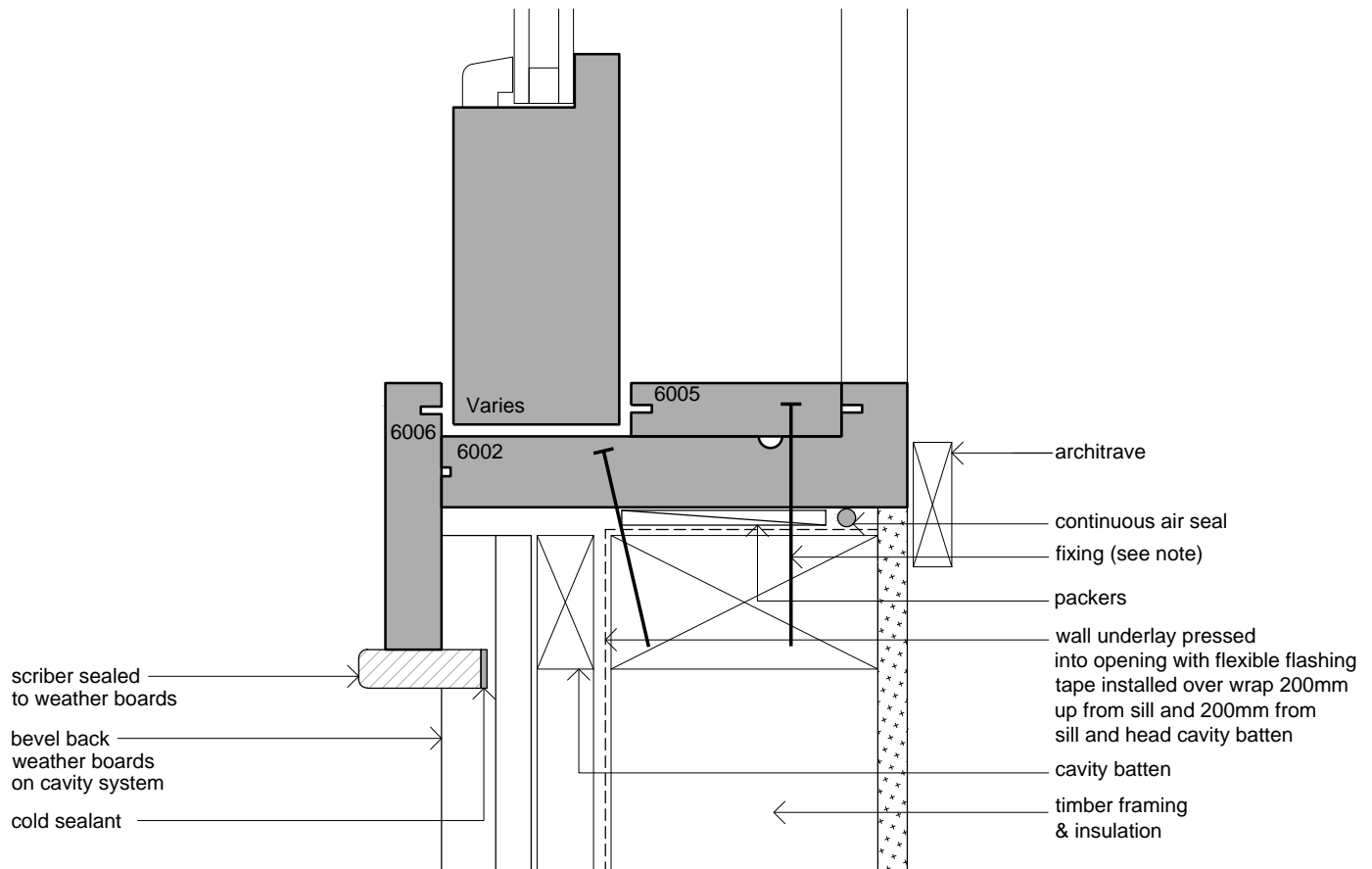
Door Jamb Scale: 1:2.5
