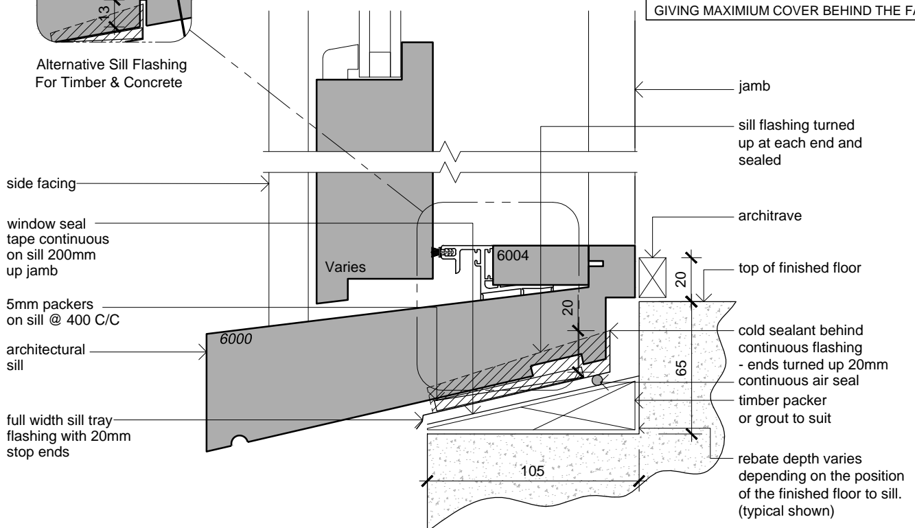
Door Sill Scale: 1:2.5
