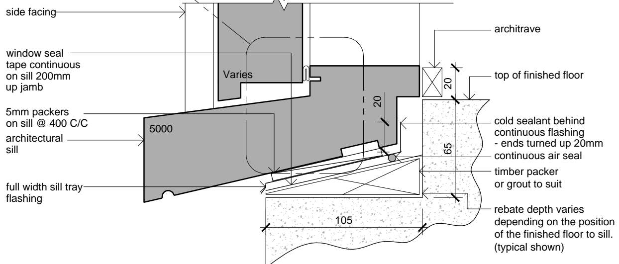
Door Sill Scale: 1:2.5
