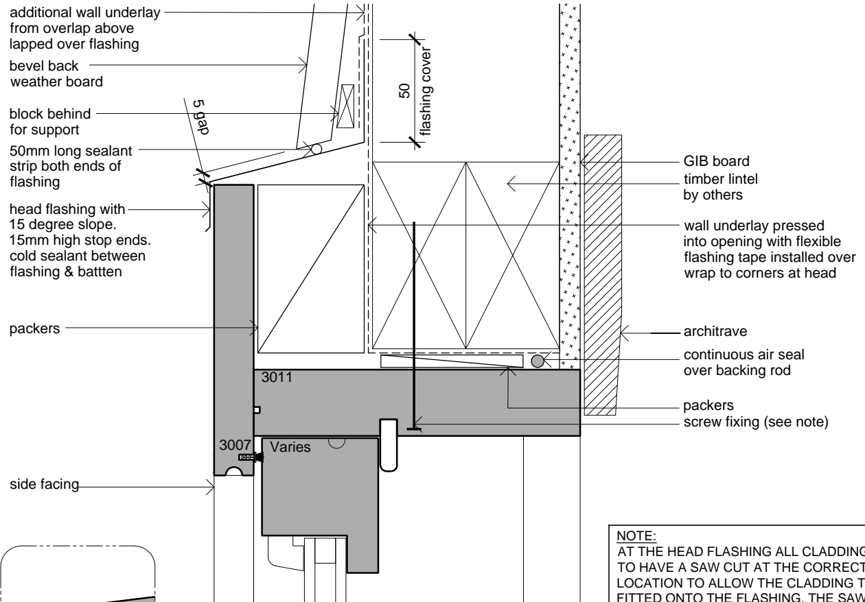
Window Head Scale: 1:2.5
