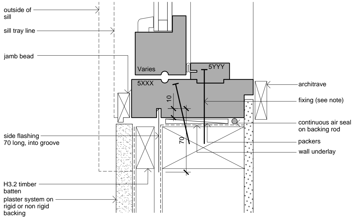
Window Jamb
