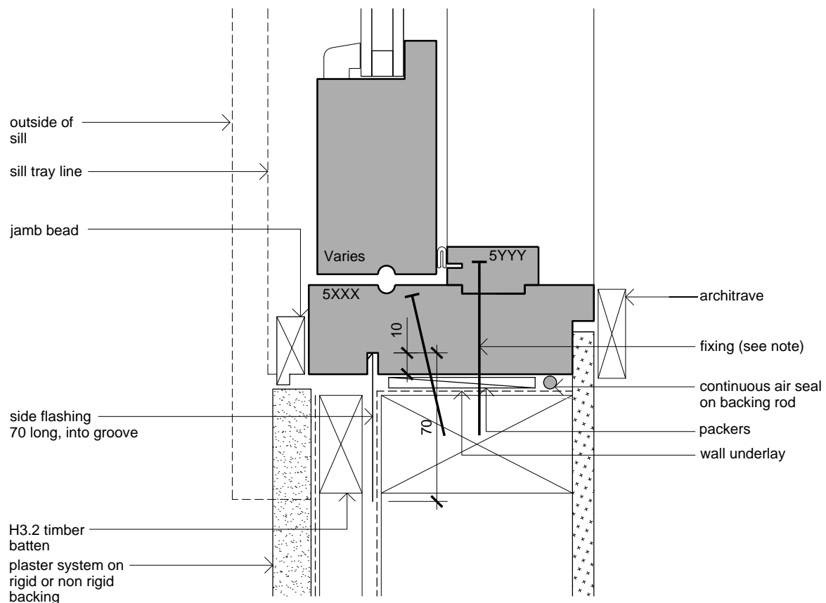
Door Jamb
