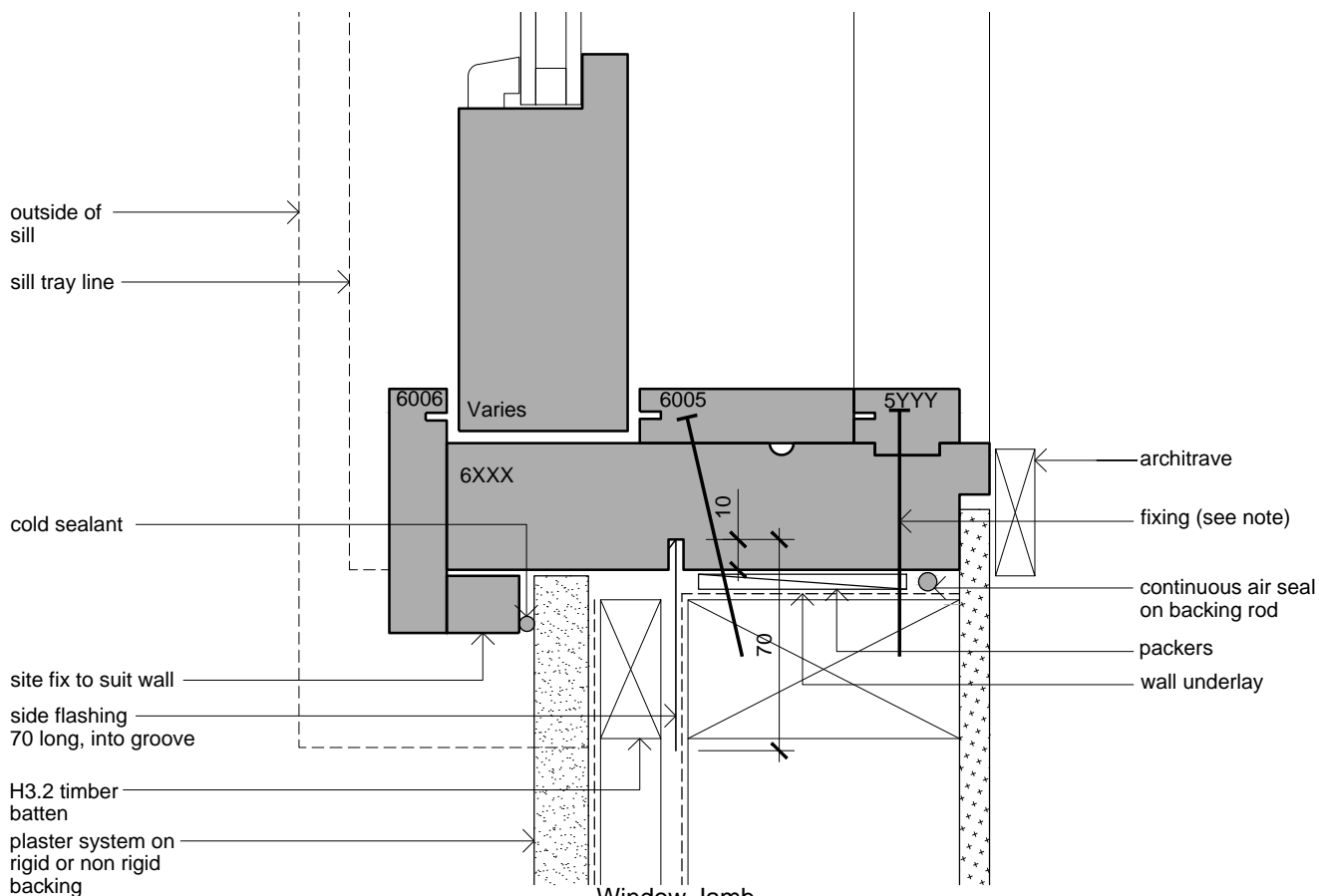
Window Jamb
