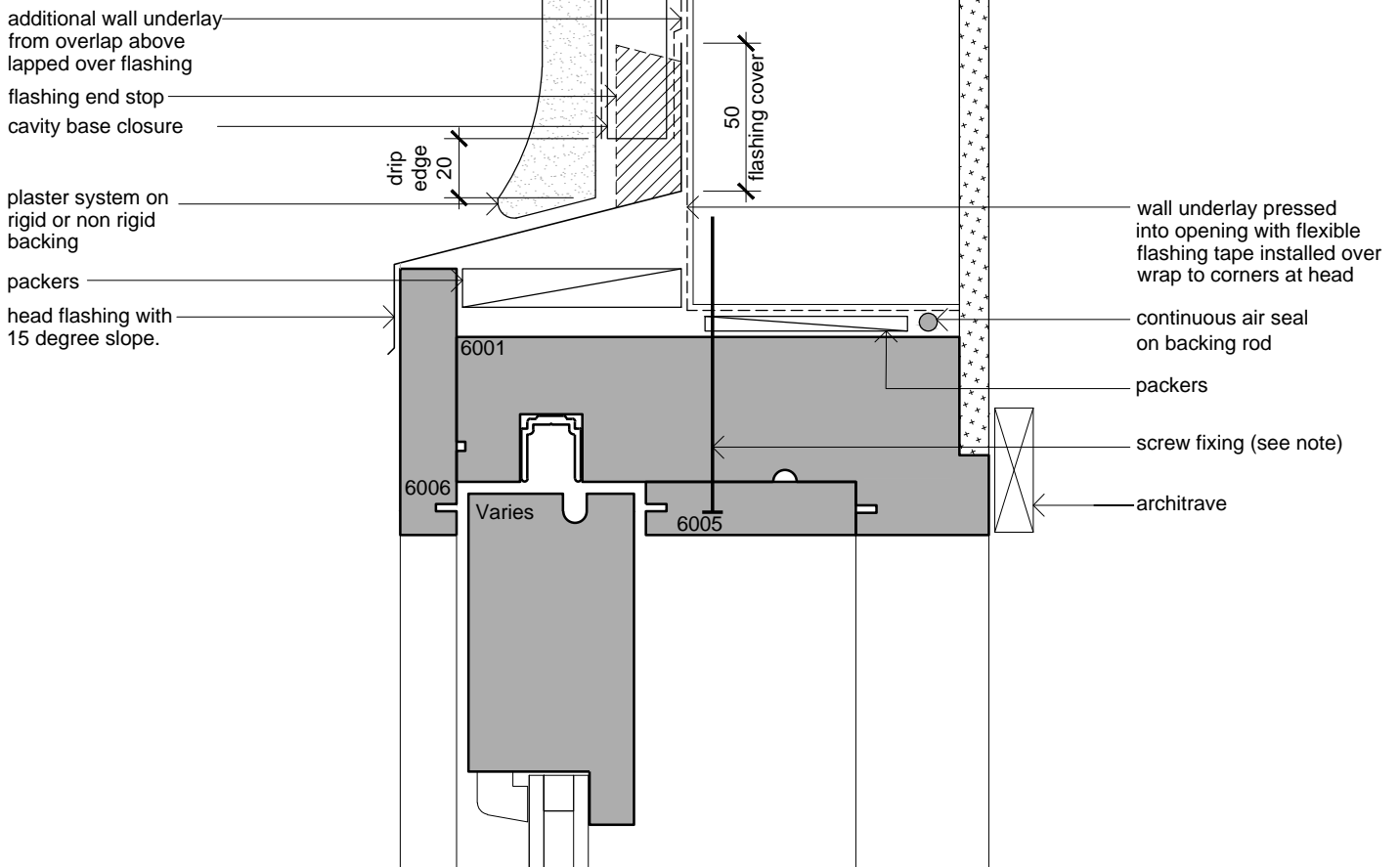
Window Head Scale: 1:2.5
