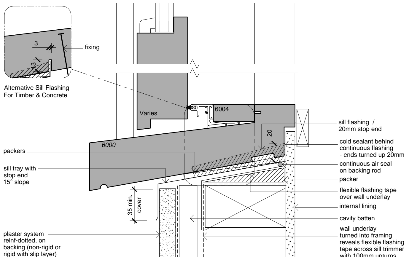
Window Sill Scale: 1:2.5
