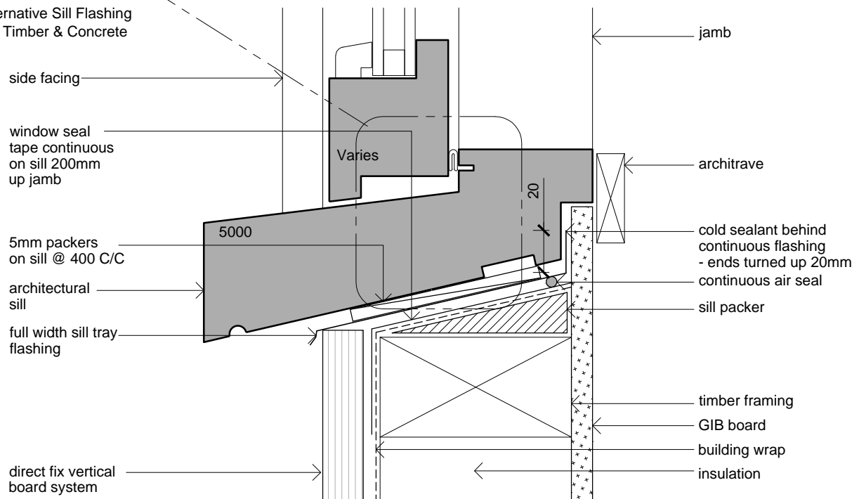
Window Sill Scale: 1:2.5
