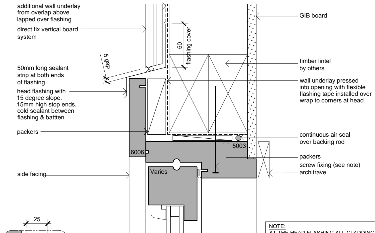
Window Head Scale: 1:2.5
