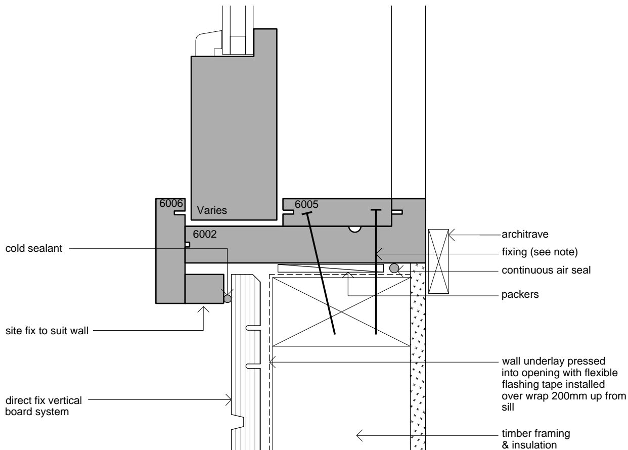
Window Jamb
