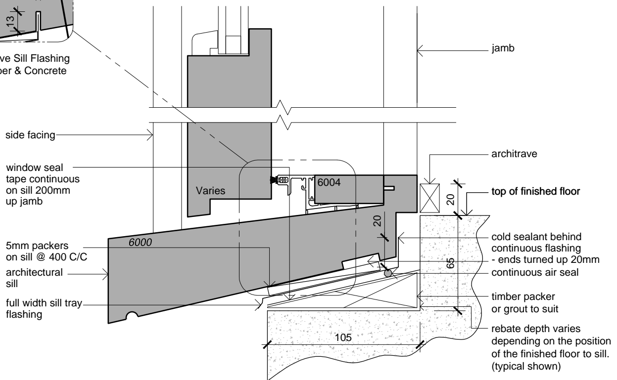
Door Sill Scale: 1:2.5
