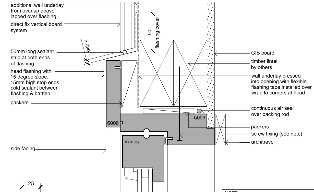
Window Head Scale: 1:2.5
