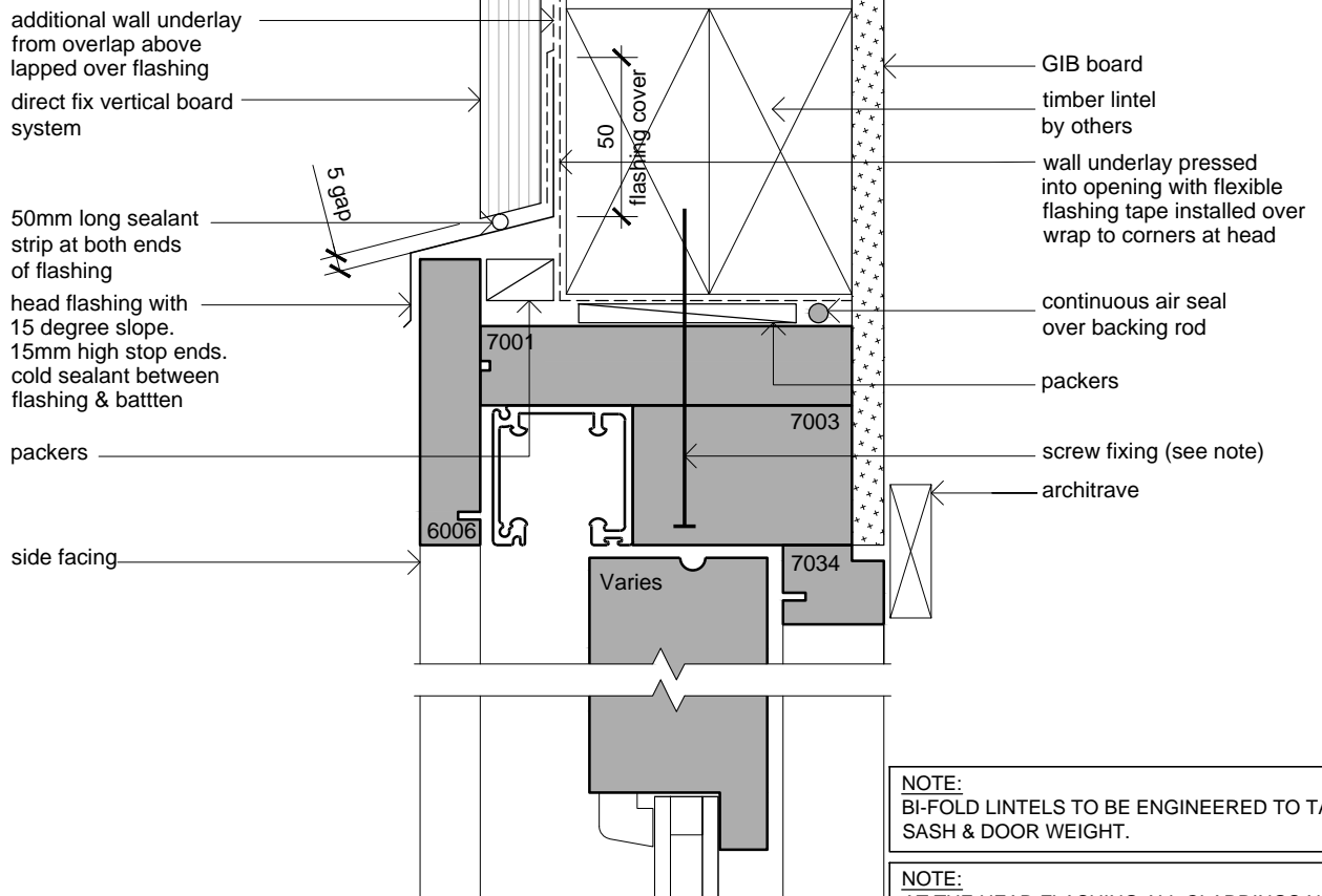
Window Head Scale: 1:2.5
