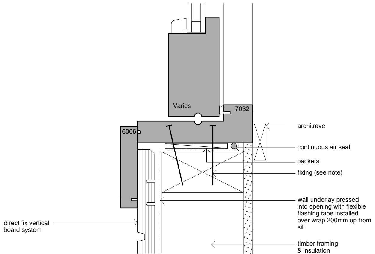
Window Jamb Scale: 1:2.5
