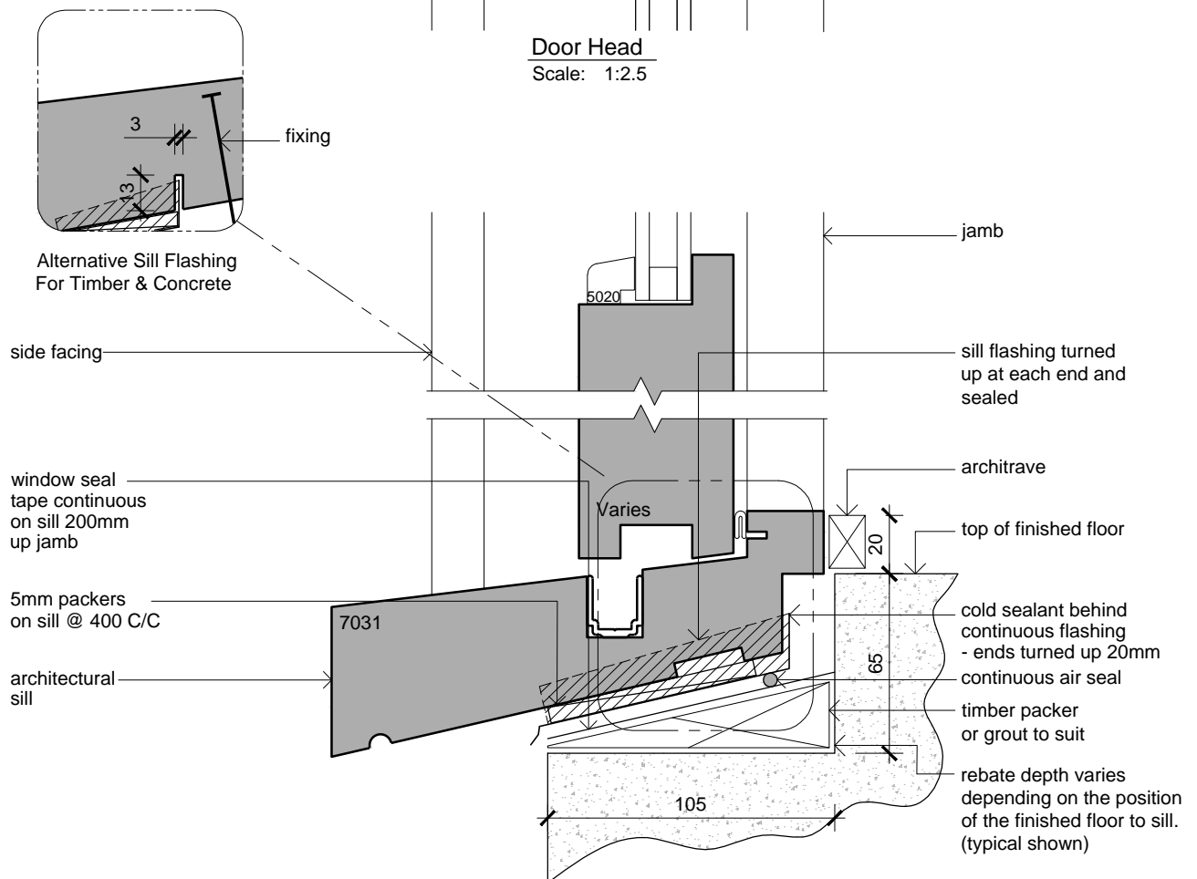
Door Sill Scale: 1:2.5
