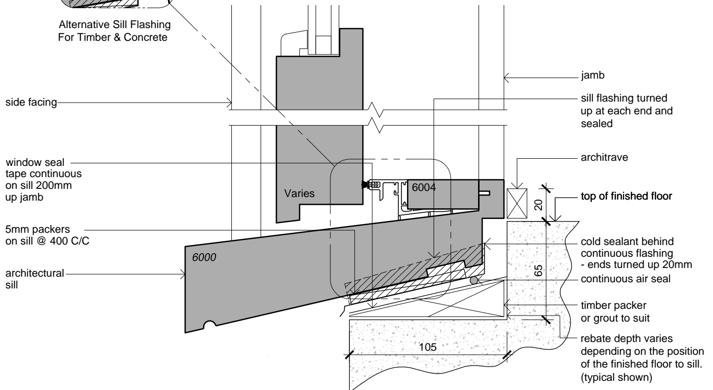
Door Sill Scale: 1:2.5
